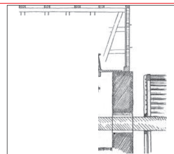
Schematischer Schnitt durch den mittelalterlichen „Untertrieb“ und das „Mahlwerk“ einer „unterschlächtigen“ Mühle, wie wir es auch für die Schwerter Mühle um 1550 voraussetzen dürfen.
